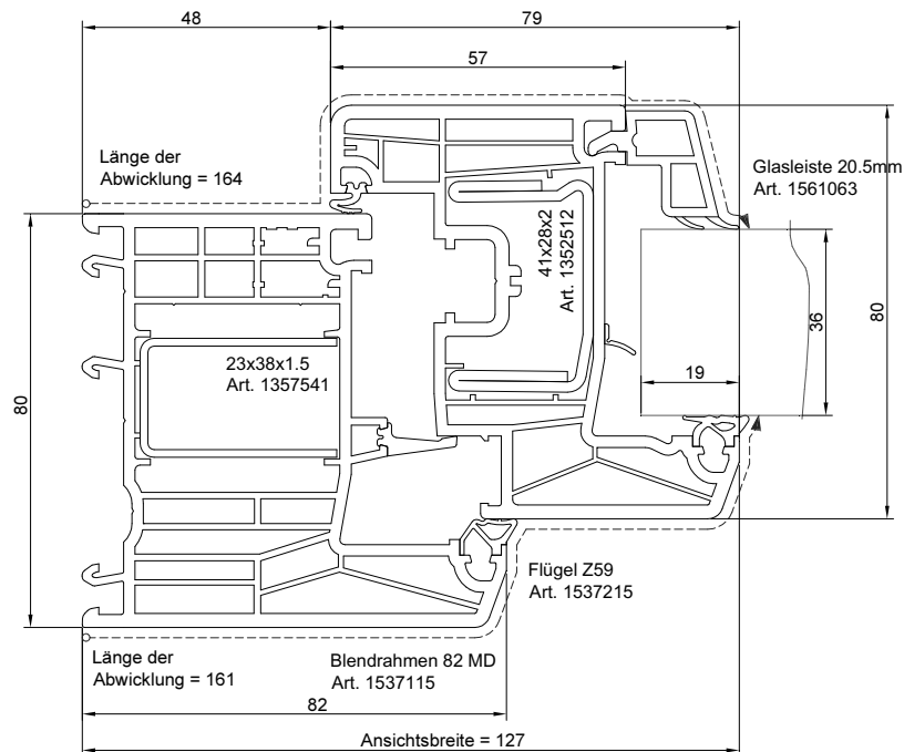
Bild 2: Querschnittsdarstellung Probekörper PK02
