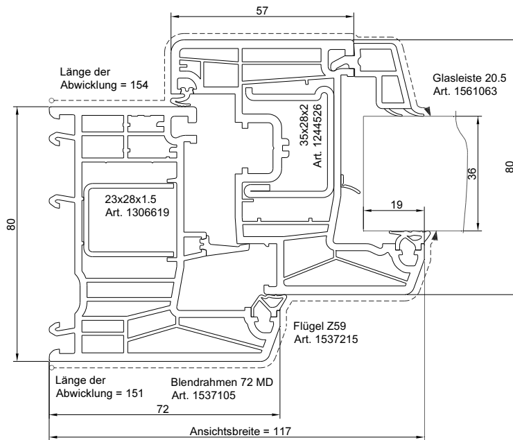
Bild 5: Querschnittsdarstellung Probekörper PK05
