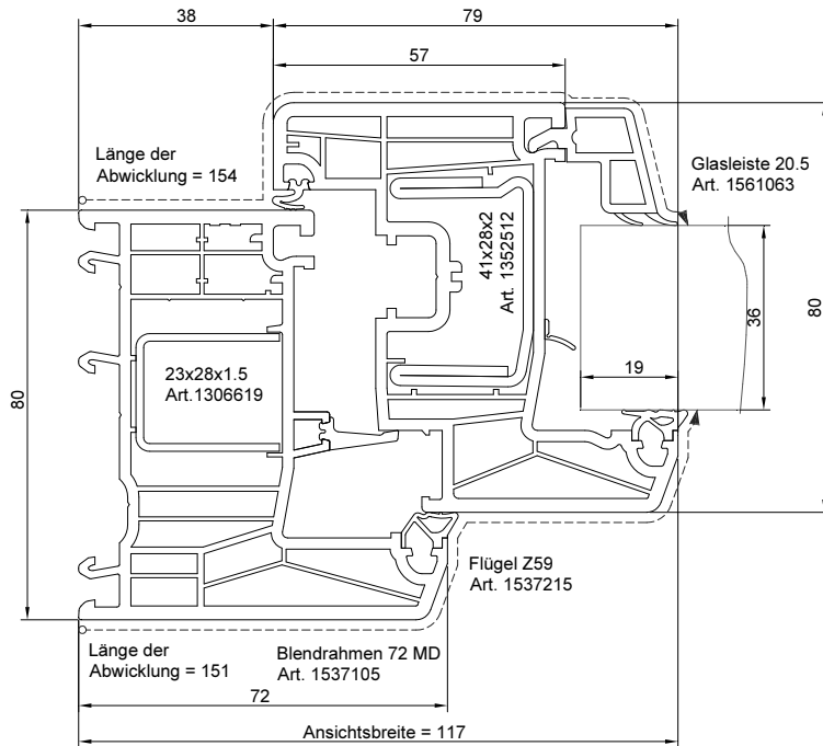
Bild 1: Querschnittsdarstellung Probekörper PK01
