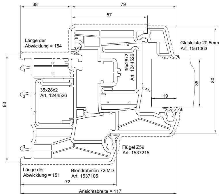
Bild 4: Querschnittsdarstellung Probekörper PK04
