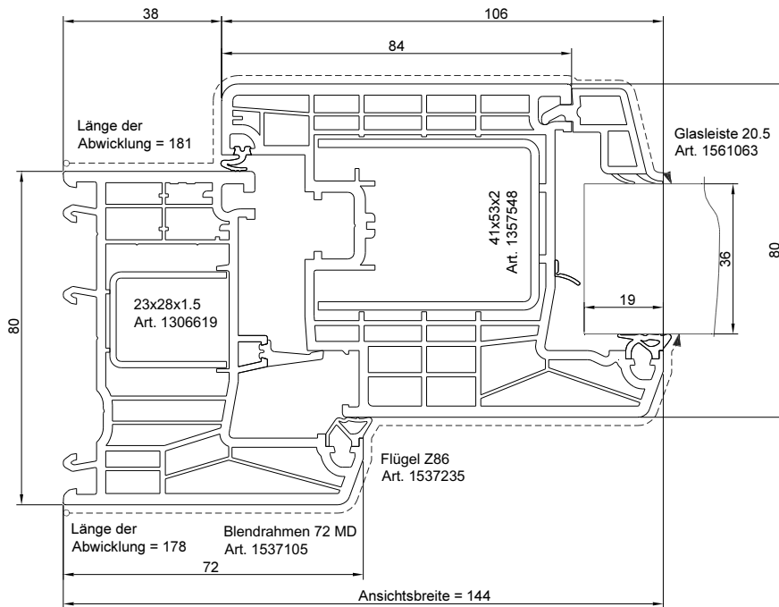
Bild 3: Querschnittsdarstellung Probekörper PK03
